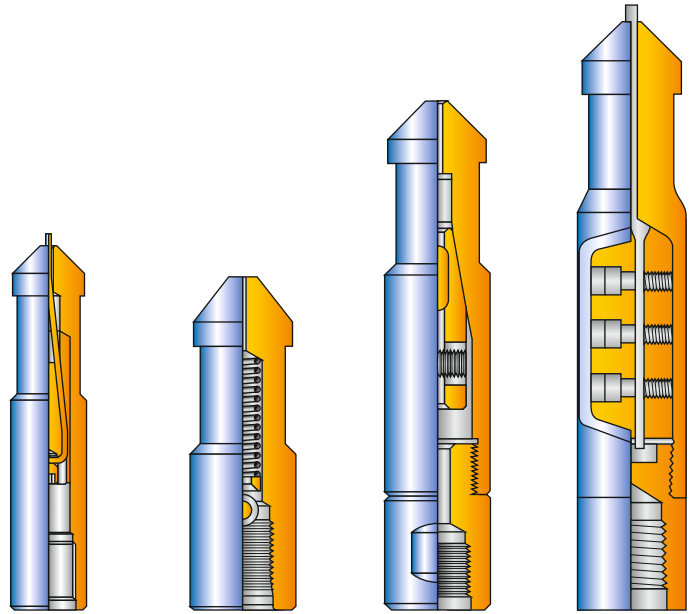
WEDGE TYPE SPOOL TYPE SLIP TYPE CLAMP TYPE
